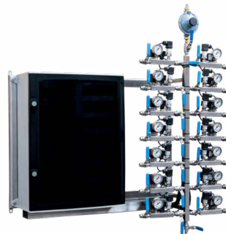
PAINEL CONTROLADOR DE NITROGÊNIO PARA SUÇO INTEGRAL
